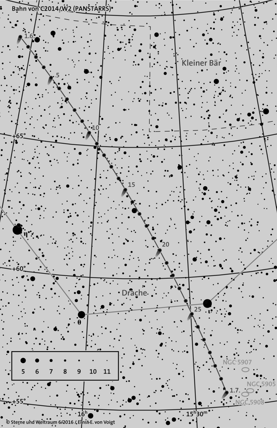
Bahn von C2014/W2 (PANSTARRS)
