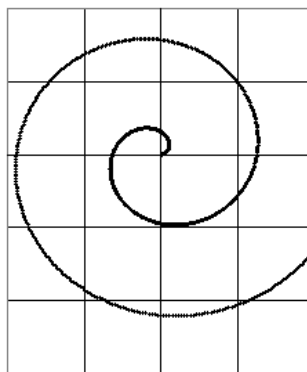
ARCHIMEDISCHE Spirale
