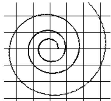
Logarithmische Spirale
