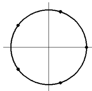
Lösungen von x^5 = 1
