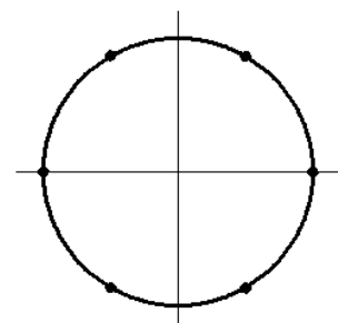
Lösungen von x^6 = 1
