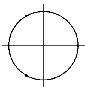
Lösungen von x^3 = 1
