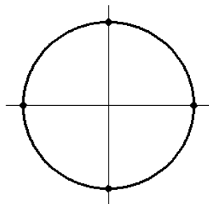
Lösungen von x^4 = 1
