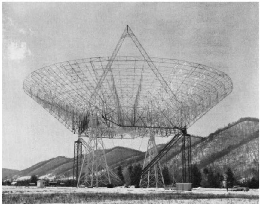
Schon 1959 hat man am US-National Radio Observatory in Green Bank mit einer speziellen Empfangsapparatur unter dem Namen „Projekt Ozma“ versucht — ohne Erfolg zwar — aus der Richtung einiger „verdächtiger“ Sterne Radiosignale zu beobachten. — Ein neues Radioteleskop von 90 m Antennen-Durchmesser ist nun im Bau, es wird sicherlich auch für die Suche nach Radiosignalen eingesetzt werden.
