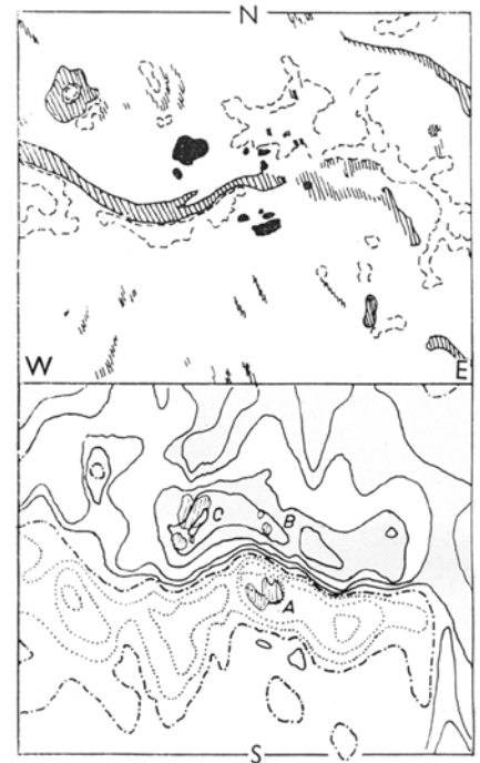
Abb. 2: Obere Karte: Die Chromosphäre im Aktivitätszentrum. Untere Karte: Verteilung der magnetischen Feldstärken.
