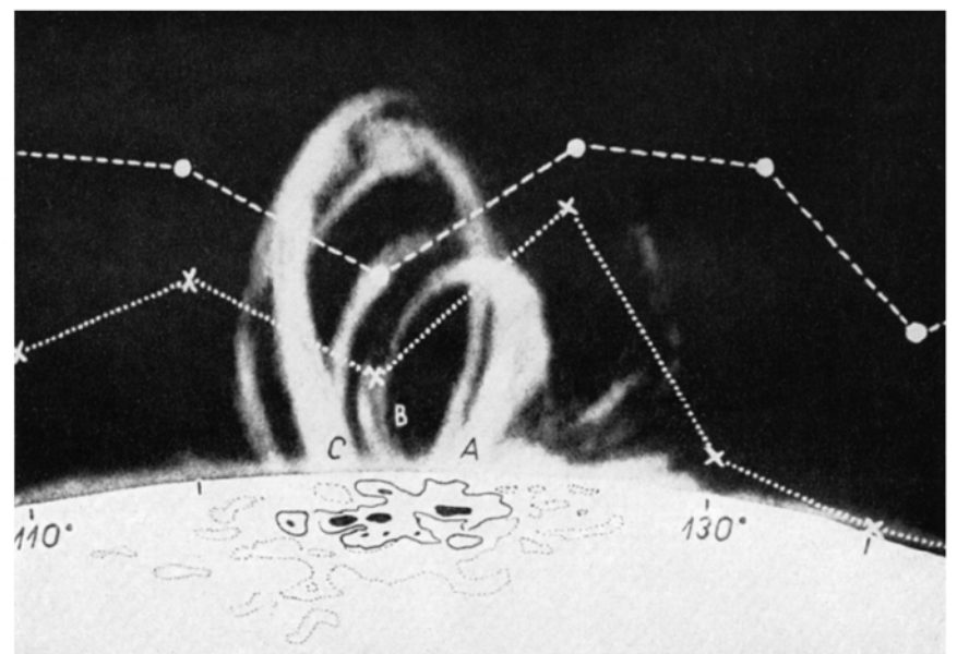
Abb. 1: Das Aktivitätszentrum am Rand der Sonnenscheibe mit Protuberanzen, Fackelgebieten und Sonnenflecken. In die Photographie sind die Intensitäten der grünen und roten Koronalinien eingezeichnet.
