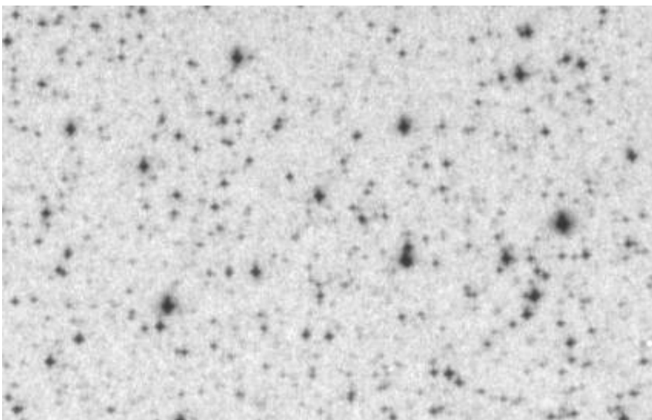
Platte 72 (300298) JD=2439379,48
