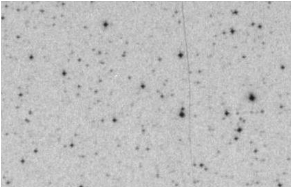
Platte 62 (300278) JD=2439200,30
