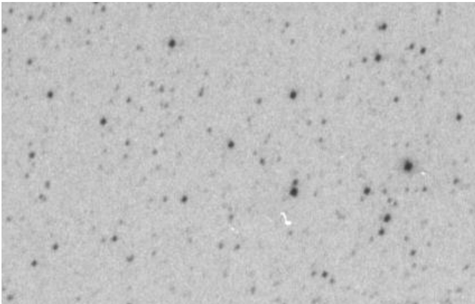
Platte 83 (300324) JD=2439593,59
