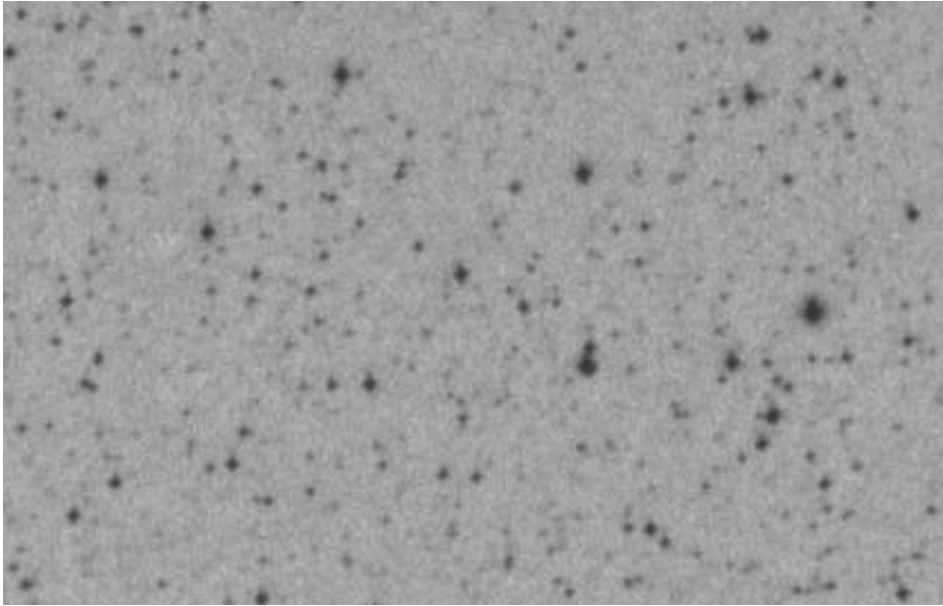
Platte 79 (300316) JD=2439508.45
