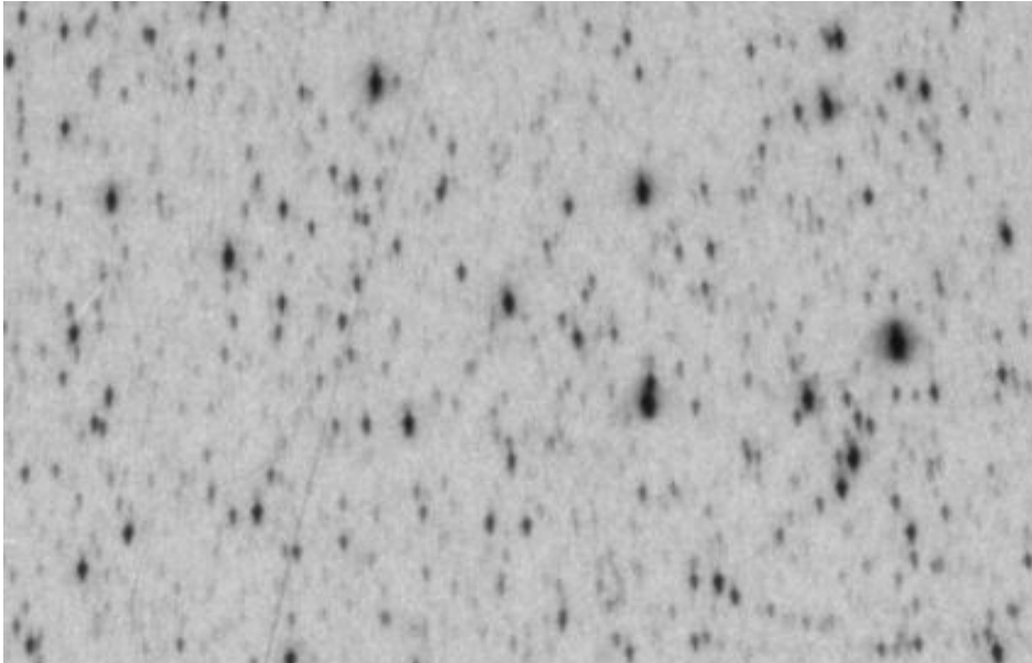
Platte 61 (300276) JD=2439146,33
