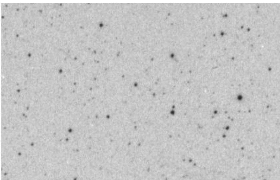
Platte 66 (300286) JD=2439286,50
