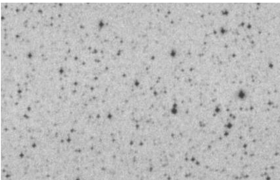
Platte 78 (300315) JD=2439500,34
