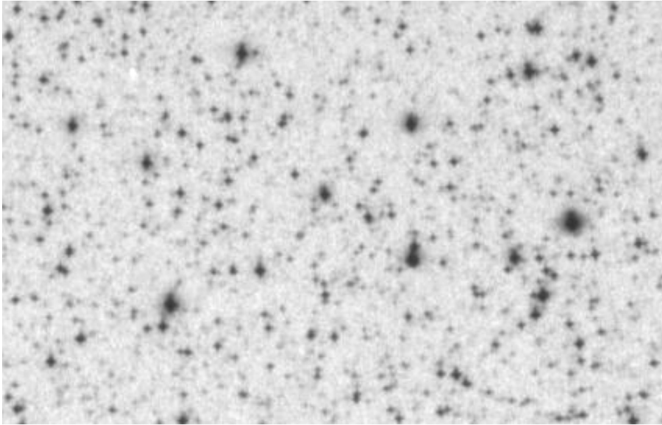
Platte 73 (300300) JD=2439385,47
