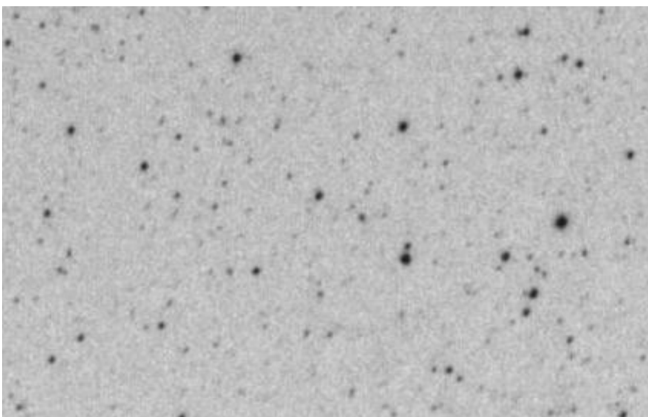
Platte 63 (300283) JD=2439242,58
