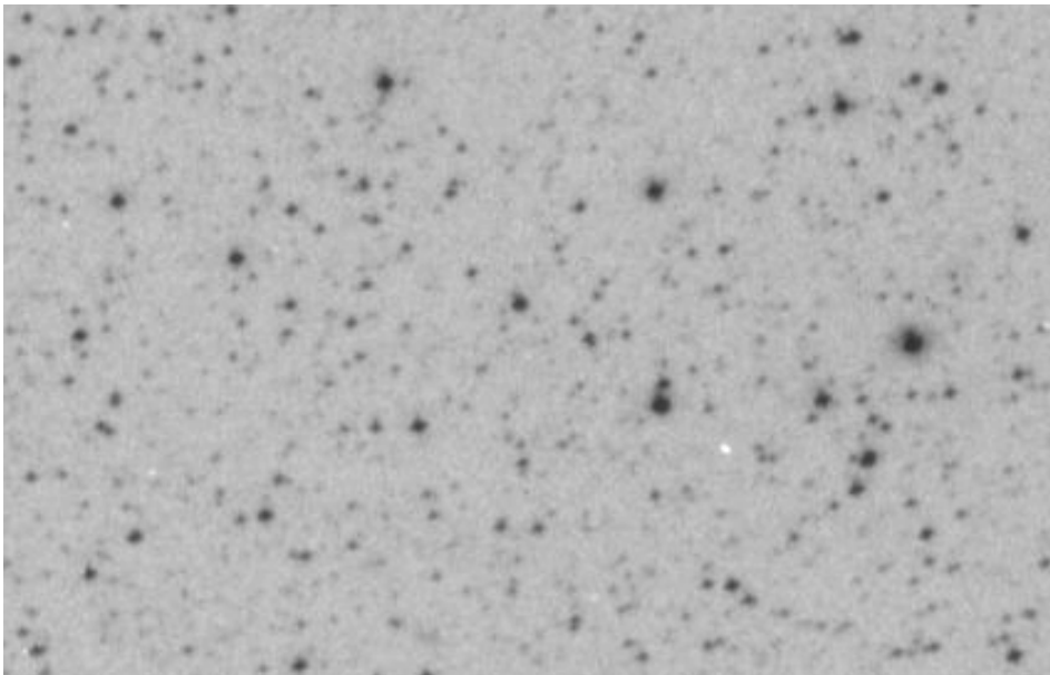
Platte 80 (300317) JD=2439521,27
