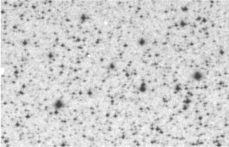
Platte 70 (300292) JD=2439350,55
