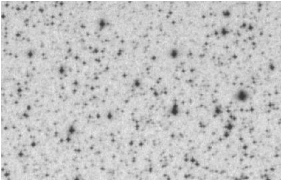
Platte 74 (300307) JD=2439406,35
