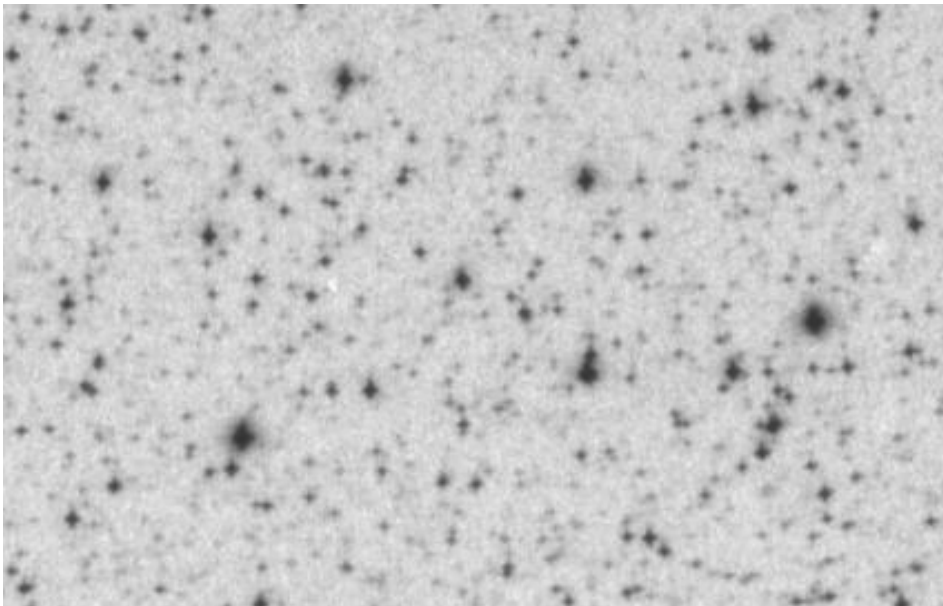
Platte 71 (300296) JD=2439359,45
