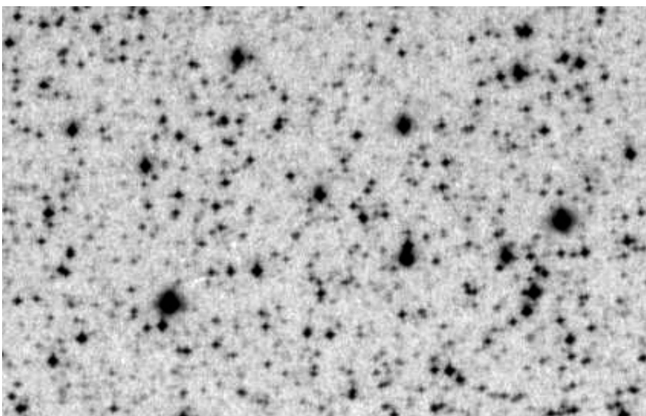
Platte 69 (300290) JD=2439330,51
