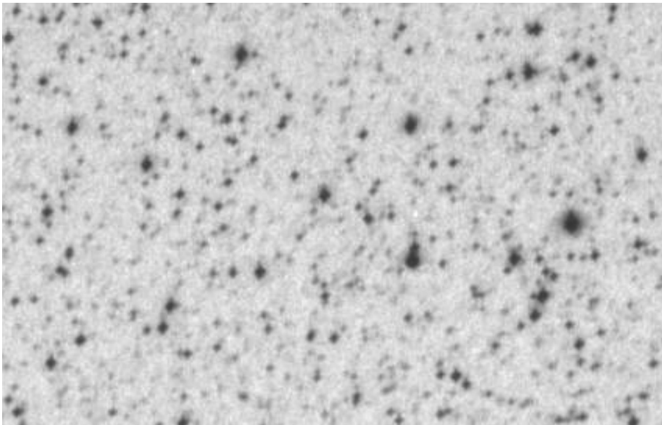
Platte 77 (300313) JD=2439442,49
