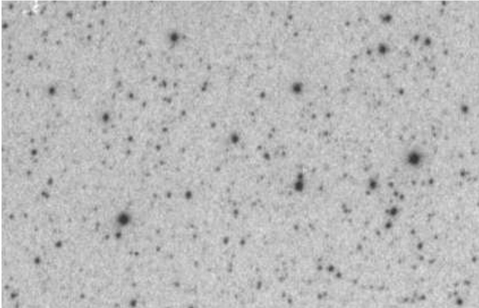
Platte 67 (300287) JD=2439299,51
