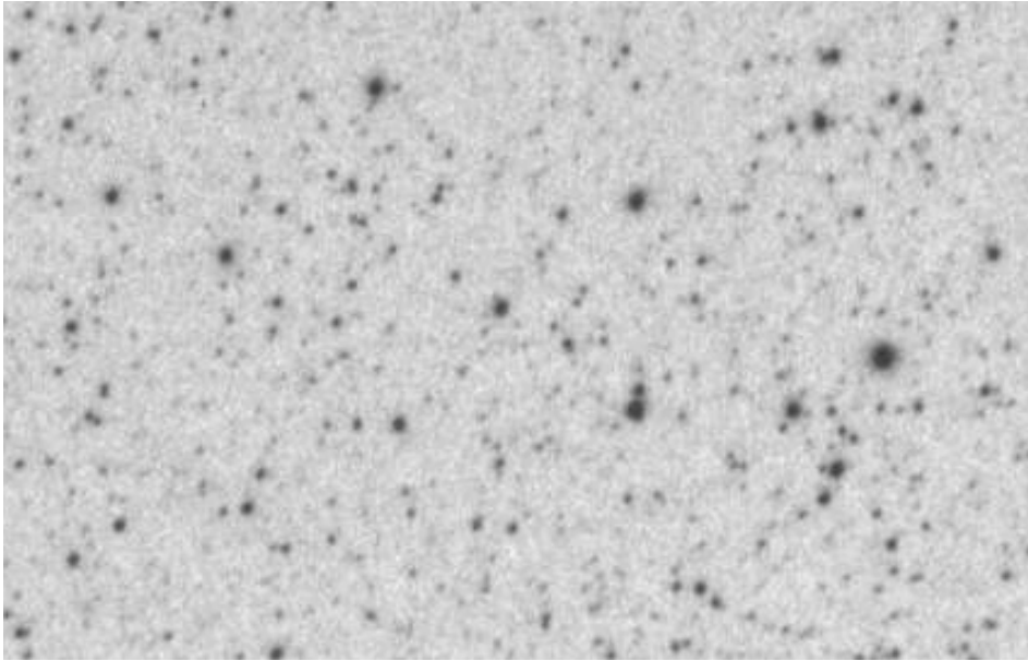
Platte 64 (300284) JD=2439263,54
