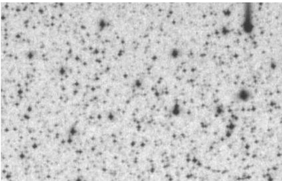
Platte 75 (300308) JD=2439413,34
