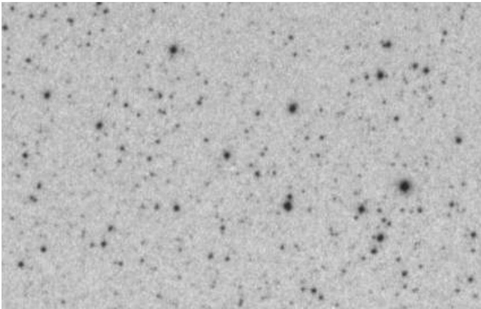
Platte 65 (300285) JD=2439270,54
