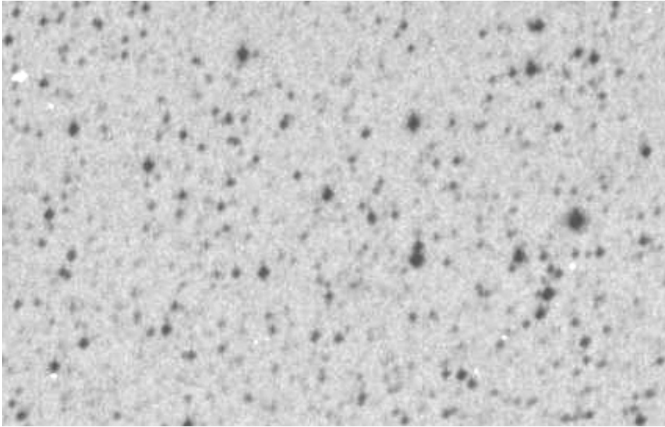
Platte 82 (300320) JD=2439533,33
