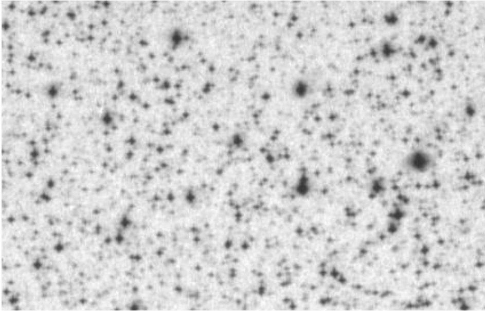
Platte 76 (300311) JD=2439436,34
