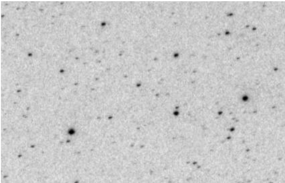
Platte 68 (300288) JD=2439317,45
