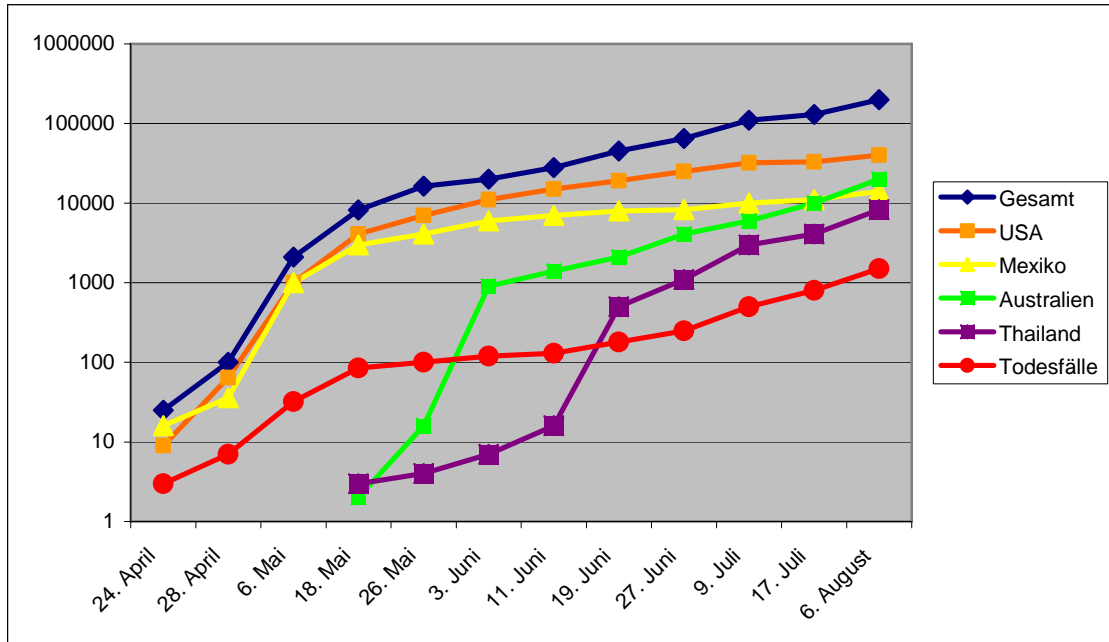
InfluenzaA (H1N1)-Fälle bei der Pandemie 2009 (Eigene Grafik verändert nach: http://www.who.int/csr/ )
